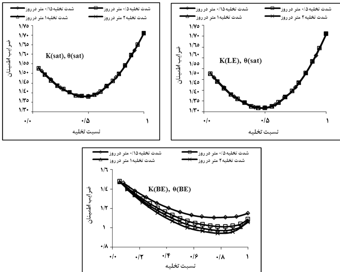
شکل ۱۰- ضرایب اطمینان تحلیل استاتیکی در مقابل نسبت تخلیه با اعمال چهار نوع شدت تخلیه متفاوت
