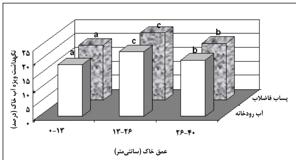
شکل ۴- اثر کیفیت آب بر نگهداشت ویژه آب خاک در عمق‌های مختلف خاک
