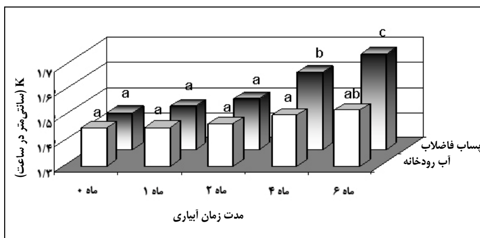
شکل ۱- اثر کیفیت آب بر ضریب هدایت هیدرولیکی اشباع خاک در مدت زمان‌های مختلف آبیاری (ستون‌های دارای حرف مشترک در سطح احتمال ۵ درصد اختلاف معنی‌داری ندارند)
