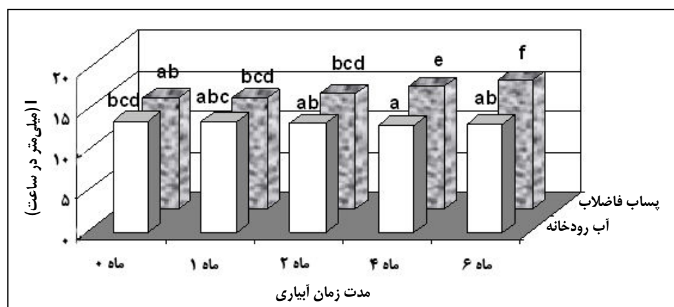
شکل ۵- اثر کیفیت آب بر نفوذپذیری نهایی لایه سطحی خاک در مدت زمان‌های مختلف آبیاری
