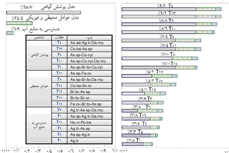
شکل 7- نمودار تحلیل حساسیت پویا وزن تیپ‌های گیاهی نسبت به سه شاخص پوشش گیاهی، عوامل محیطی و منابع آب
