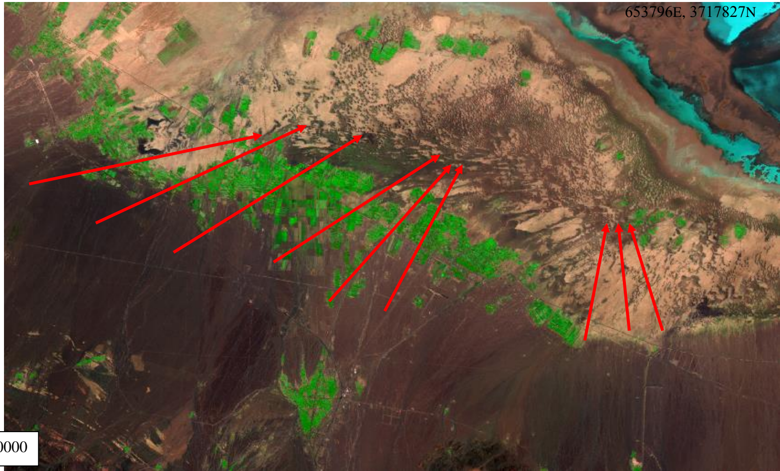
شکل 2- تصویر ترکیب کاذب رنگی RGB742 در منطقه مطالعاتی اردستان
