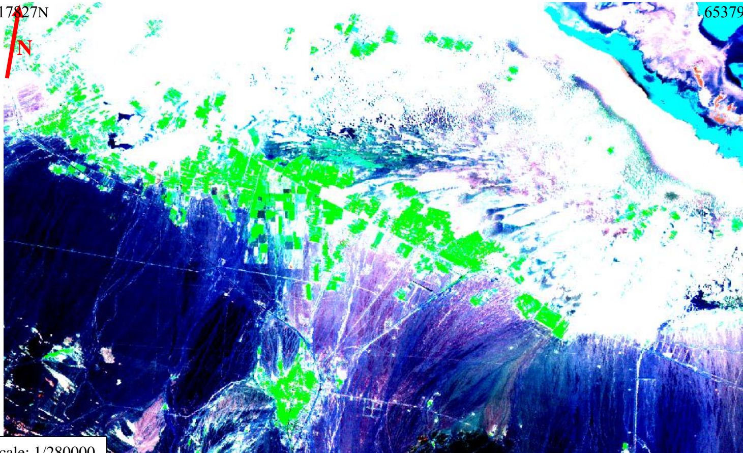
شکل 3- تصویر حاصل از افزایش تباین و روشنایی RGB742 در منطقه مطالعاتی اردستان
