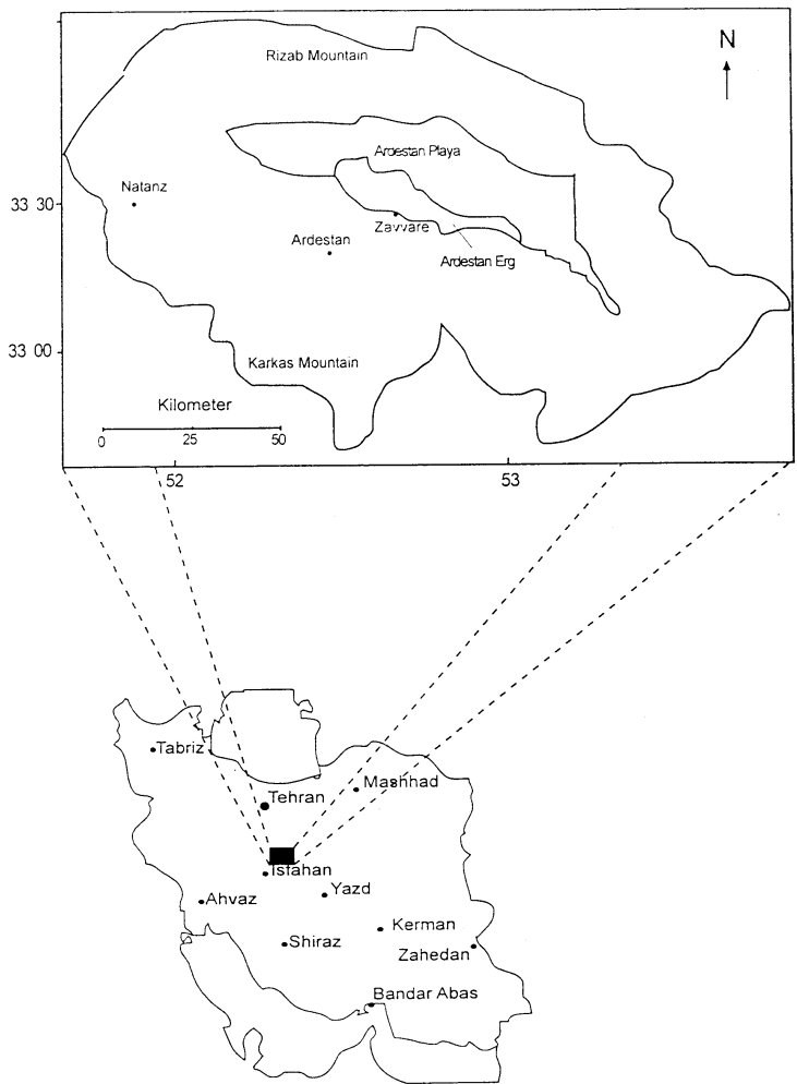
شکل 1- موقعیت منطقه مطالعاتی در کشور (اشتری مهرجردی، 1380)
