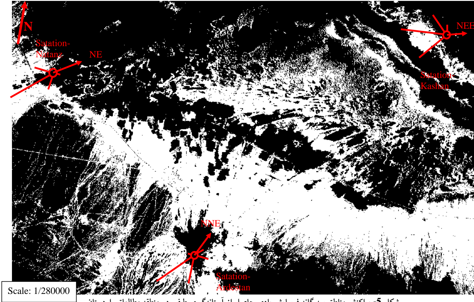
شکل 5- پراکنش مناطق سه گانه فرسایش بادی حاصل از آستانه گیری طیفی در منطقه مطالعاتی اردستان
