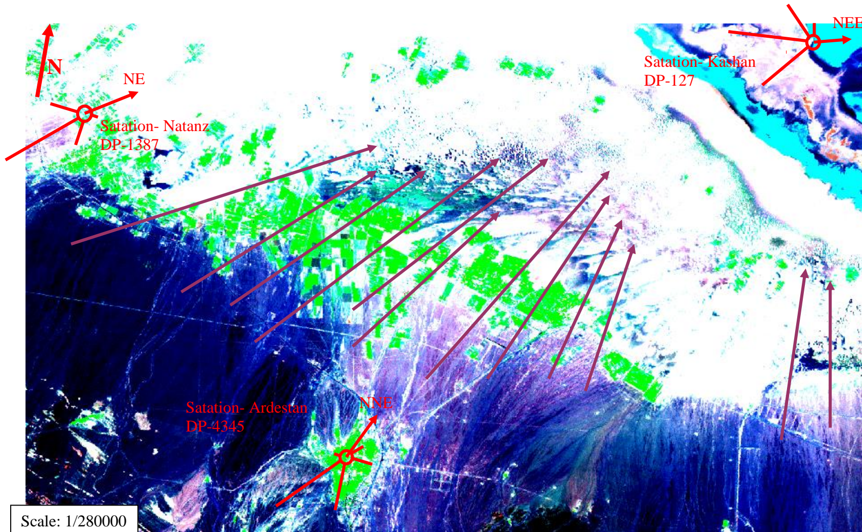
شکل 8- تصویر حاصل از افزایش تباین و روشنایی شکل 42 در منطقه مطالعاتی اردستان
