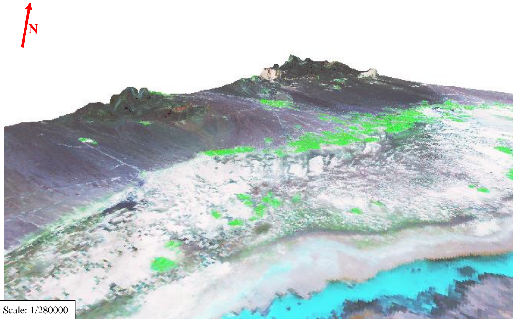
شکل 4- تلفیق تصویر حاصل از افزایش تباین و روشنایی ترکیب کاذب رنگی RGB742 و مدل ارتفاعی رقومی در منطقه مطالعاتی اردستان
