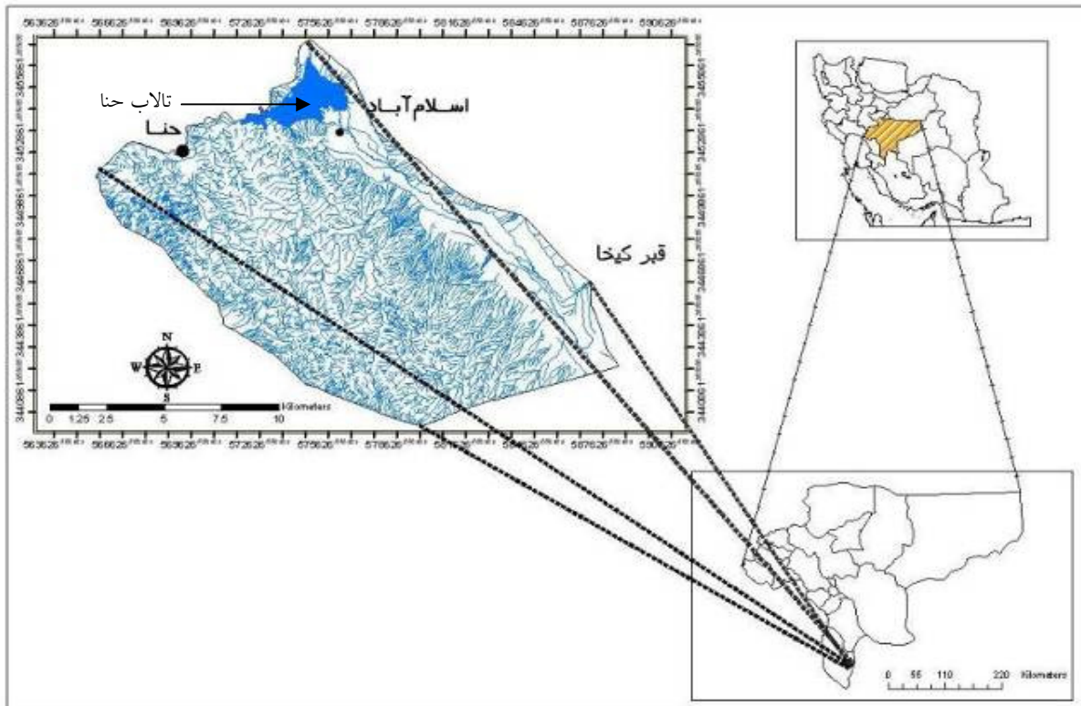
شکل ۱: موقعیت جغرافیای منطقه مورد مطالعه (اقتباس از محبوبی صوفیانی، ۱۳۸۸)
