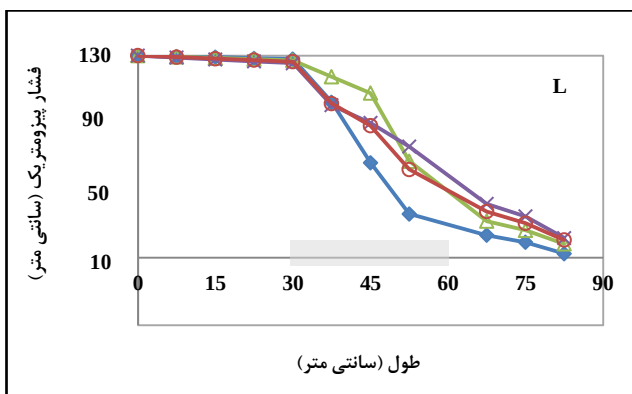
شکل ۱۲- فشار پیژومتریکی در مقابل درصدهای مختلف آهک تحت تراز ۱/۲ متر
