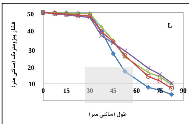
شکل ۸- فشار پیژومتریکی در مقابل درصدهای مختلف آهک تحت تراز ۰/۴ متر
