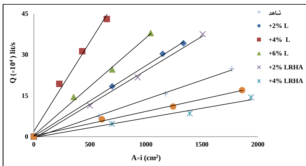
شکل ۷- دبی در مقابل A \times i برای نمونه‌های مختلف
