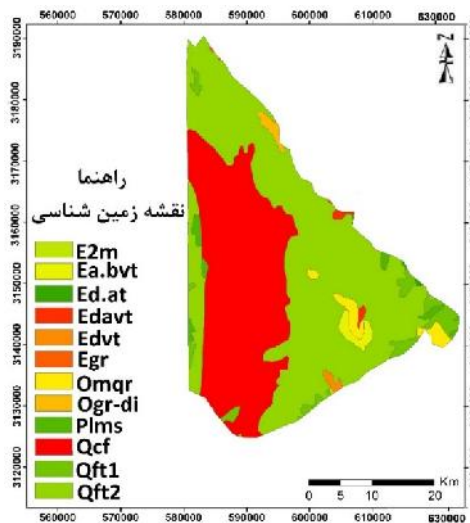
شکل ۴- نقشه زمین شناسی دشت جیرفت
