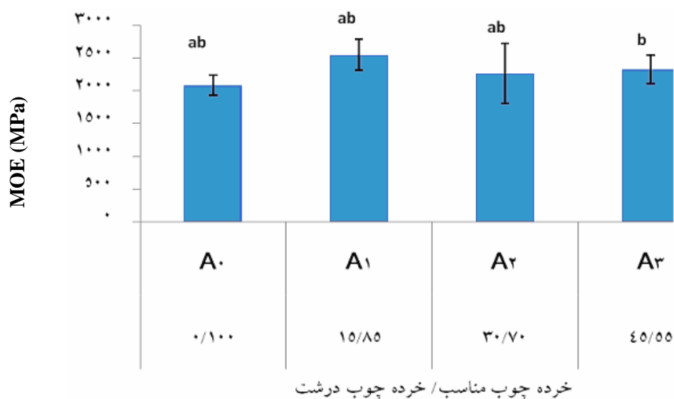
شکل ۴ - اثر مقدار خرده‌های چوب درشت بر مدول الاستیسیته تخته‌ها
