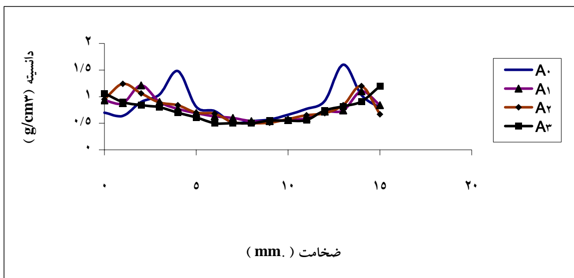
شکل ۱۰- پروفیل دانسیته تخته‌های تیمار A 0 ، A 1 ، A 2 و A r
