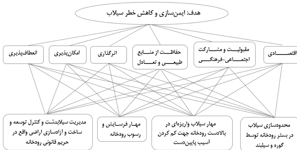
شکل ۴- سلسله مراتب تصمیم گیری با هدف ایمن سازی و کاهش خطر سیلاب
