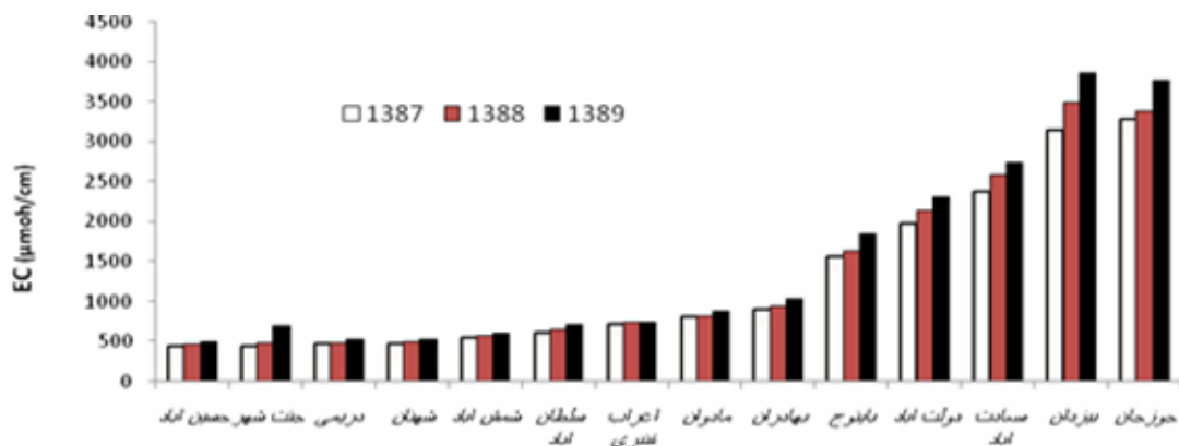
شکل ۷- تغییرات هدایت الکتریکی آب چاه مناطق مختلف دشت داراب طی سال‌های ۸۷ تا ۸۹.
