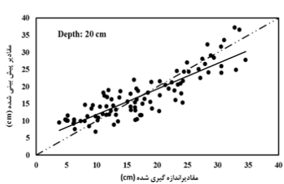
شکل ۵- مقایسه داده‌های اندازه‌گیری و برآورد شده شعاع خیس‌شده پایین قطره‌چکان هر سه عمق در اعماق مختلف با خط ۱:۱
