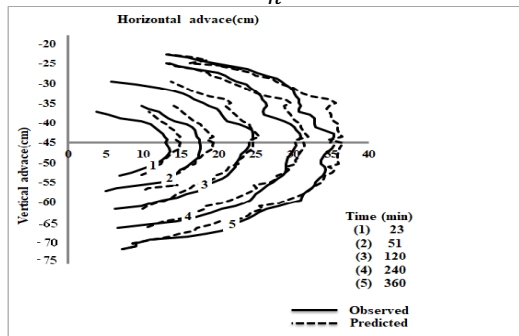
شکل ۳- پیاز رطوبتی اندازه‌گیری شده در مقایسه با مقادیر شبیه‌سازی شده در خاک لومی برای تیمارهای مختلف
