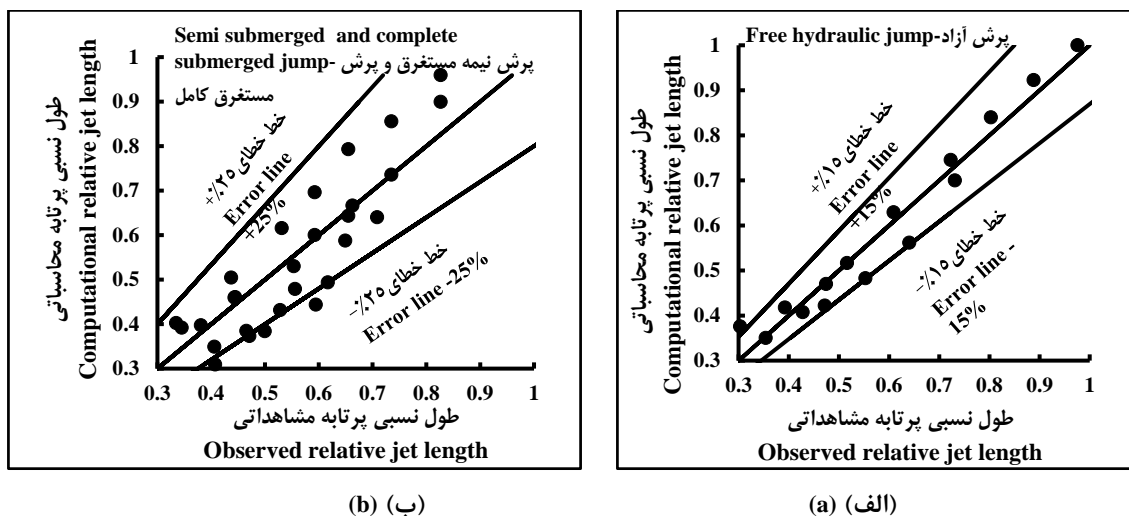
شکل ۱۶- مقایسه طول نسبی پرتابه مشاهداتی (آزمایشگاهی) و محاسباتی از رابطه ۱۵ و (ب) رابطه ۱۶ Fig. 16 - Comparison of the relative length of the observational (laboratory) and computational jet from (a) relation 15 and (b) relation 16
