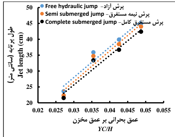
شکل ۱۴- طول پرتابه در پرتاب‌کننده با چهار دفلکتور در برابر \frac{Y_c}{H} و عمق‌های متفاوت پایاب
