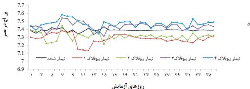
شکل ۲: نمودار تغییرات میزان اکسیژن محلول در صبح (الف)، اکسیژن محلول در عصر (ب)، pH در صبح (ج) و pH در عصر (د) تحت تاثیر تیمارها در روزهای مختلف آزمایش
