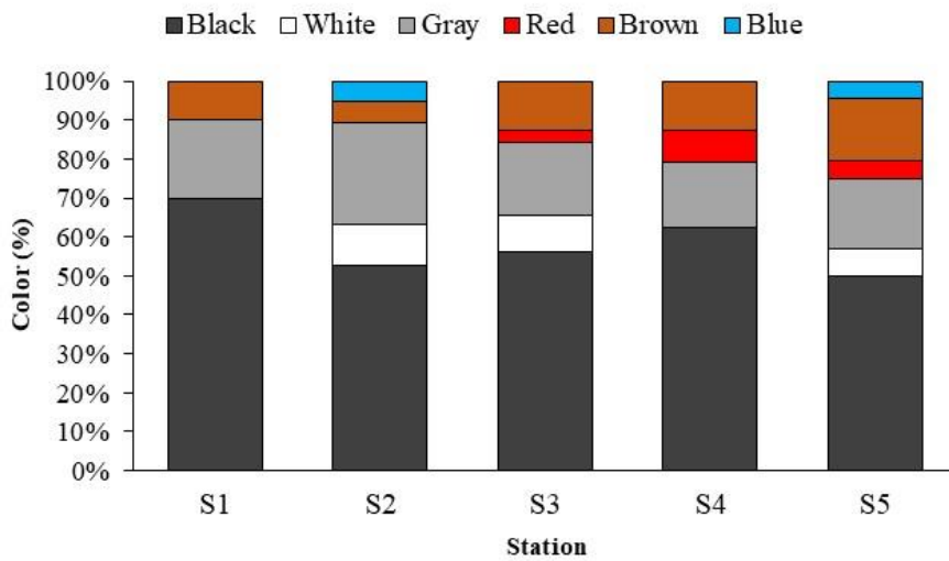
شکل ۶: درصد فراوانی رنگ میکروپلاستیک‌های استخراجی در نمونه‌های رسوب از رودخانه خرمارود Figure 6: Percentage abundance of color-microplastics extracted in sediment samples from Khormarud River
