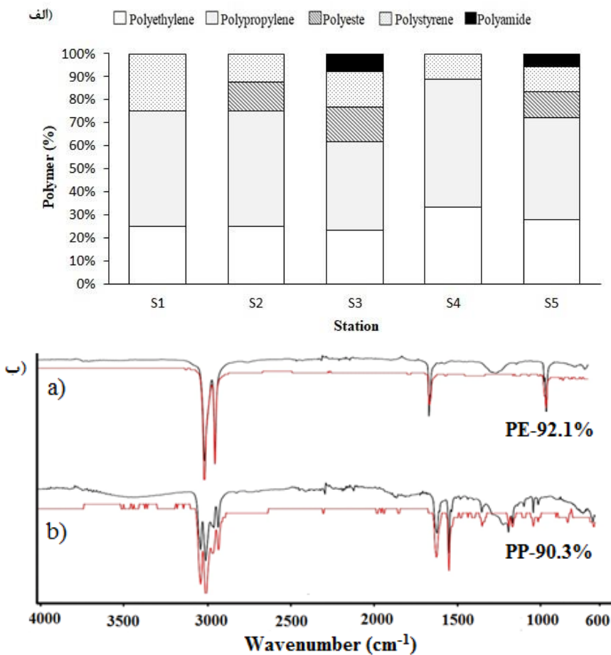
شکل ۷: الف - درصد فراوانی پلیمرهای شناسایی شده از نمونه‌های رسوبات، ب - طیف FTIR و مطابقت درجات گزیننده‌های انتخابی Figure 7: A: Percentage of abundance of polymers identified from sediment samples. B: FTIR spectrum and the degree of conformity of the selected items
