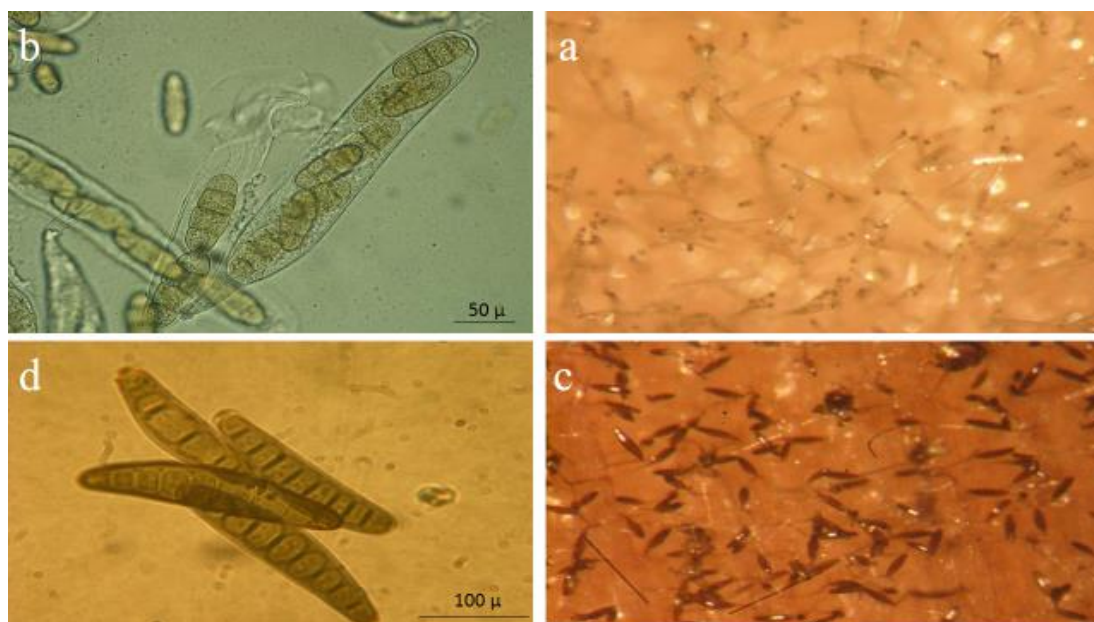
شکل ۱- اندام‌های باردهی قارچ Pyrenophora tritici-repentis (a: کنیدیوم‌های قارچ زیر بینوکولر b: تصویر میکروسکوپی آسک و آسکوسپورهای قارچ) و
