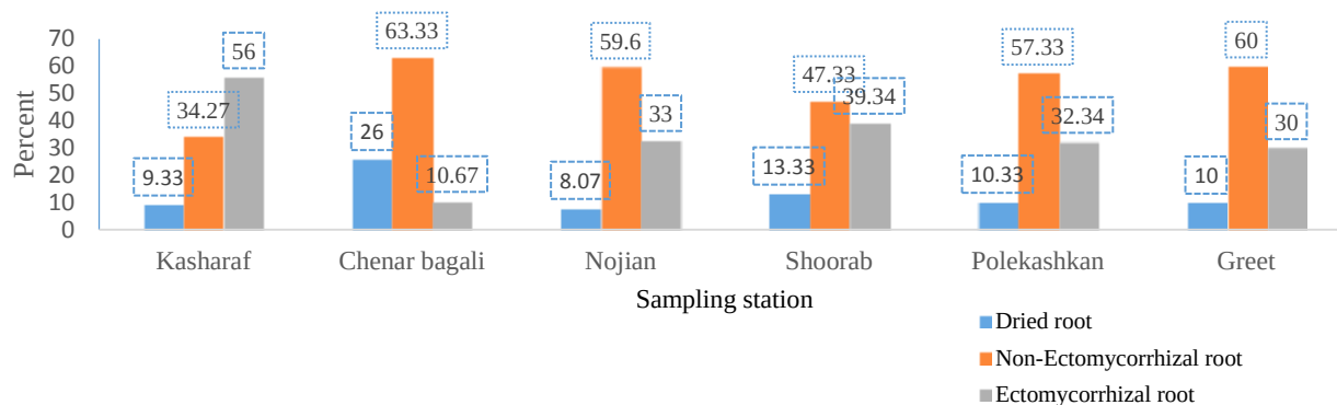
شکل ۱- مقایسه میانگین درصد ریشه‌های اکتومیکوریزایی، ریشه‌های غیراکتومیکوریزایی و ریشه‌های غیرزنده در درختان بلوط در مناطق بررسی‌شده
