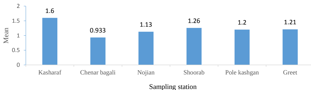
شکل ۲- مقایسه میانگین تعداد مورفوتایپ‌های اکتومیکوریزایی در درختان بلوط در مناطق نمونه‌برداری
