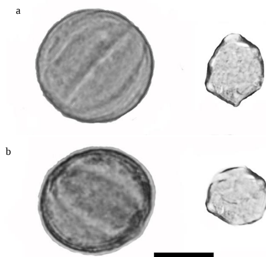
Fig. 2 The images show a fertile pollen grain on the left and a sterile pollen grain on the right. a: N. racemosa ; b: N. pungens .
