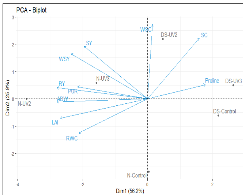
شکل ۱۱ بای پلات حاصل از گروه‌بندی تیمار و صفات مورد بررسی در چغندر قند
