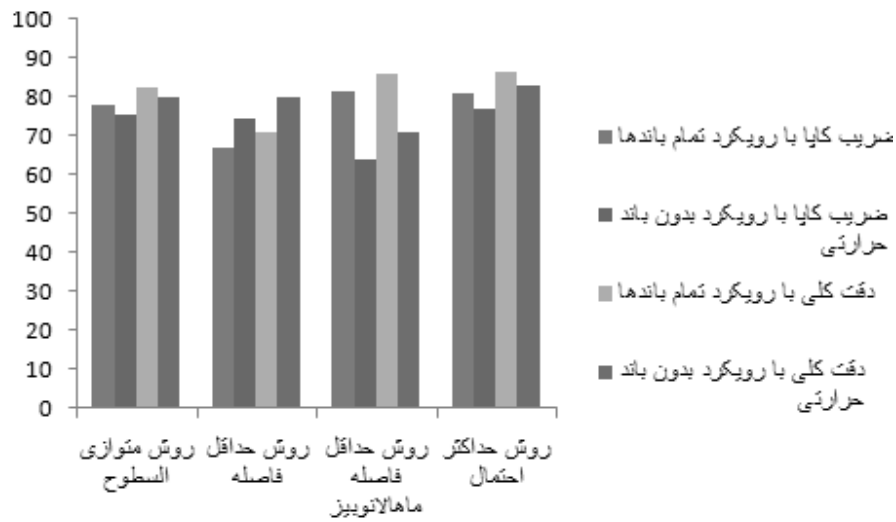
شکل ۳- مقایسه ضرب کاپا با صحت کلی سنجنده TM با رویکرد تمام باندها و رویکرد بدون باند حرارتی
