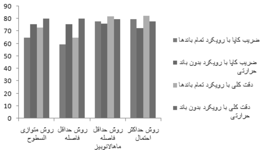
شکل ۴- مقایسه ضرب کاپا با صحت کلی سنجنده ETM+ با رویکرد تمام باندها و رویکرد بدون باند حرارتی
